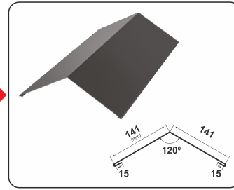
КУТОВИЙ ГРЕБІНЬ
