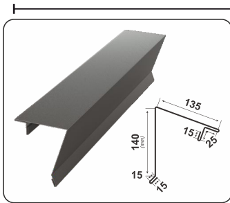
НАПІВГРЕБІНЬ RETRO
