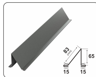
СНІГОЗАТРИМУВАЧ
