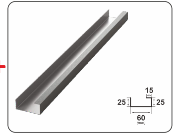
ОПОРА ГРЕБНЯ
