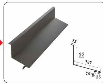
ВЕРТИКАЛЬНА ТОРЦЕВА ПЛАНКА RETRO
