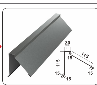
КУТОВИЙ НАПІВГРЕБІНЬ
