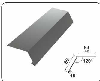
КАРНИЗНА ПЛАНКА
