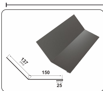
РОЗРИВ СКАТА УВІГНУТИЙ
