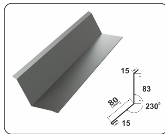
ТОРЦЕВА ПЛАНКА
