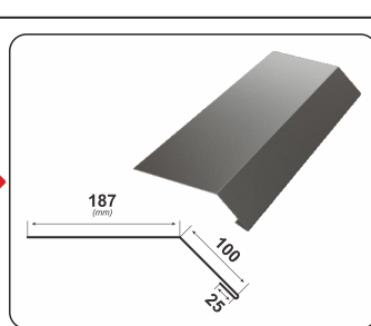
РОЗРИВ СКАТА ОПУКЛИЙ
