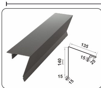
POLOVIČNÝ HREBENÁČ RETRO
