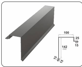
ŠTÍTOVÁ OBRUBA RETRO
