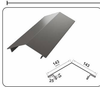
HREBENÁČ RETRO
