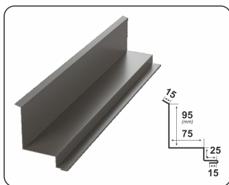
LEMOVANIE BOČNEJ STENY RETRO
