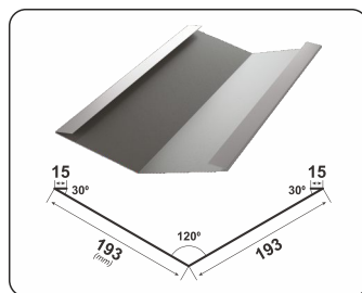
ÚŽĽABIE RETRO
