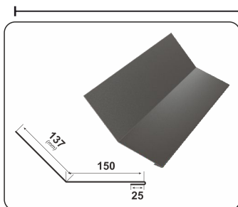
ZMENA SKLONU KONKÁVNA
