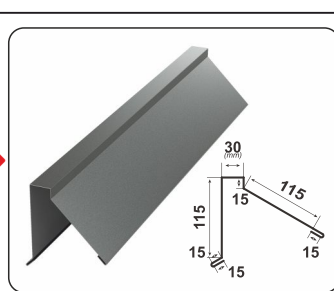
UHLOVÝ POLOVIČNÝ HREBENÁČ
