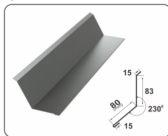
BOČNÉ LEMOVANIE
