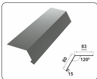
LEMOVANIE STRECHY
