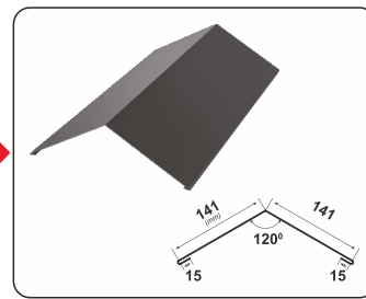
UHLOVÝ HREBENÁČ
