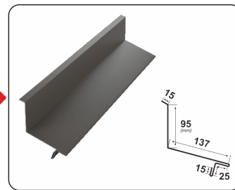
OTOK ŚCIENNY RETRO
