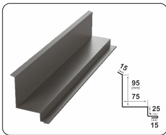
OTOK ŚCIENNY BOCZNY RETRO
