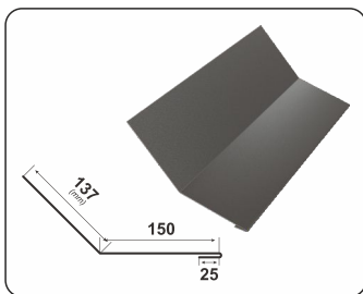
ZAŁAMANIE NACHYLENIA WKŁĘŚLE
