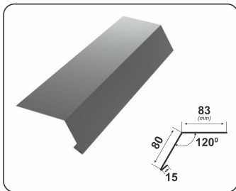
OTOK CIENIA OPADOWEGO
