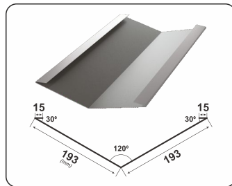
KOSZ DACHU RETRO
