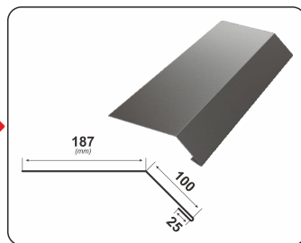
ZAŁAMANIE NACHYLENIA WYPUKŁĘ
